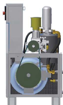
Sistema di tensionamento automatico della cinghia
