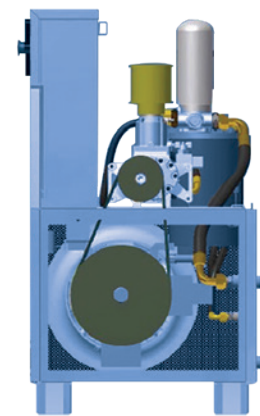
Tension automatique de la courroie
